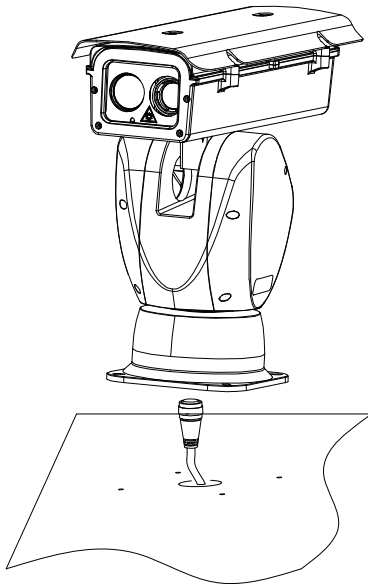
台面安装钻攻图
