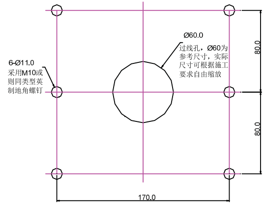
壁装钻攻图
