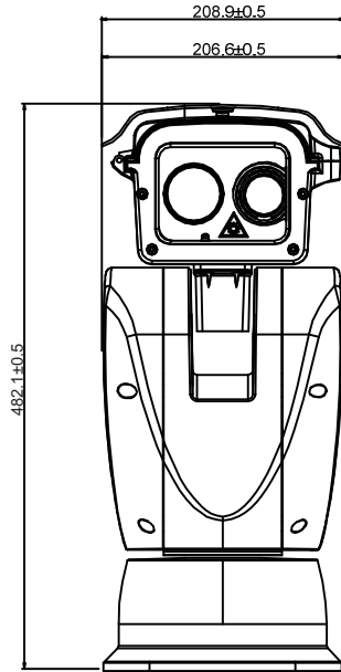
云台正视
