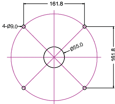
台面安装钻攻图
