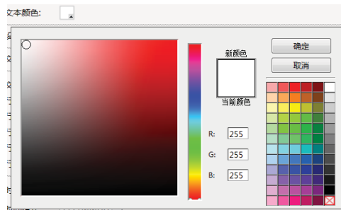
图 4-43 文本颜色
