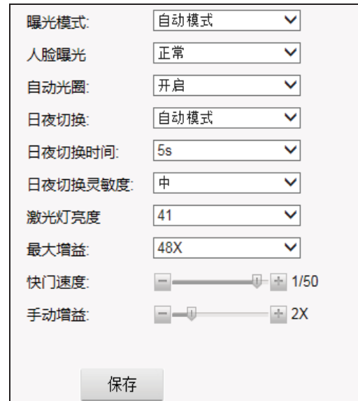
图 4-36 曝光设置
