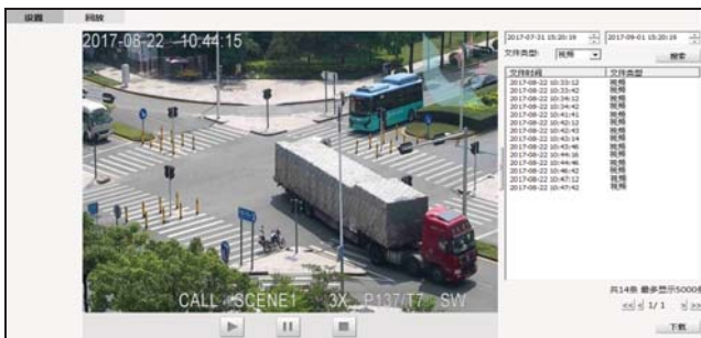
图 4-67 搜索视频
