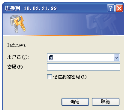
图 4-1 登录对话框
