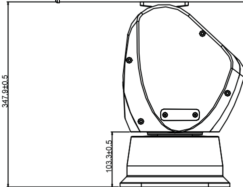
云台侧视 (18寸护罩)
