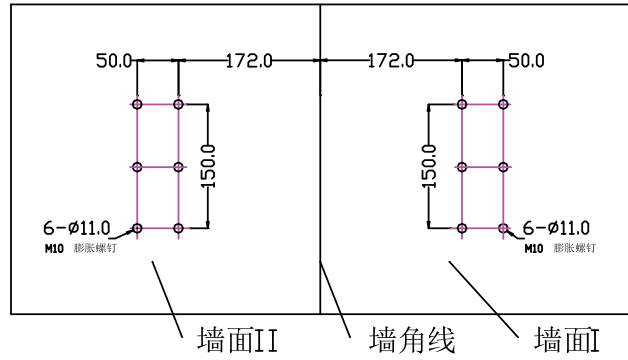
角装适配器钻攻图
