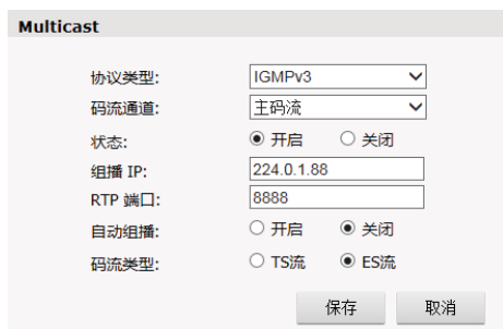
图 4-19 Multicast 设置
