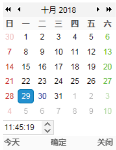
图 4-78 时间设置
