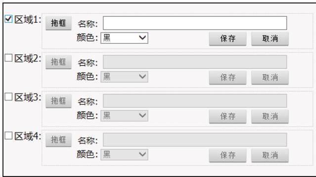
图 4-44 隐私设置
