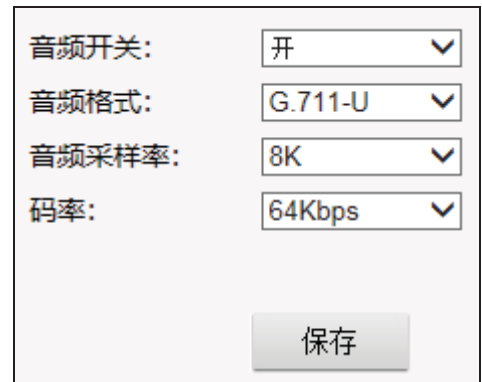
图 4-47 音频设置
