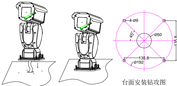
云台底部走线（主要用于下面空间充足的台面安装）
