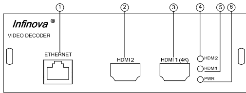
前面板图
