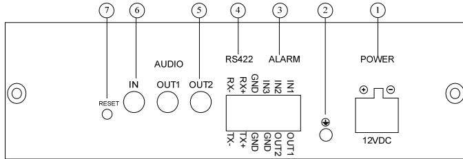
后面板图
